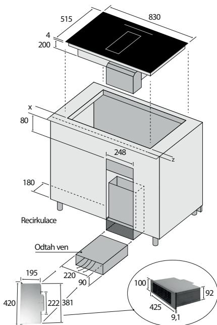
Instalace v rovině s deskou
